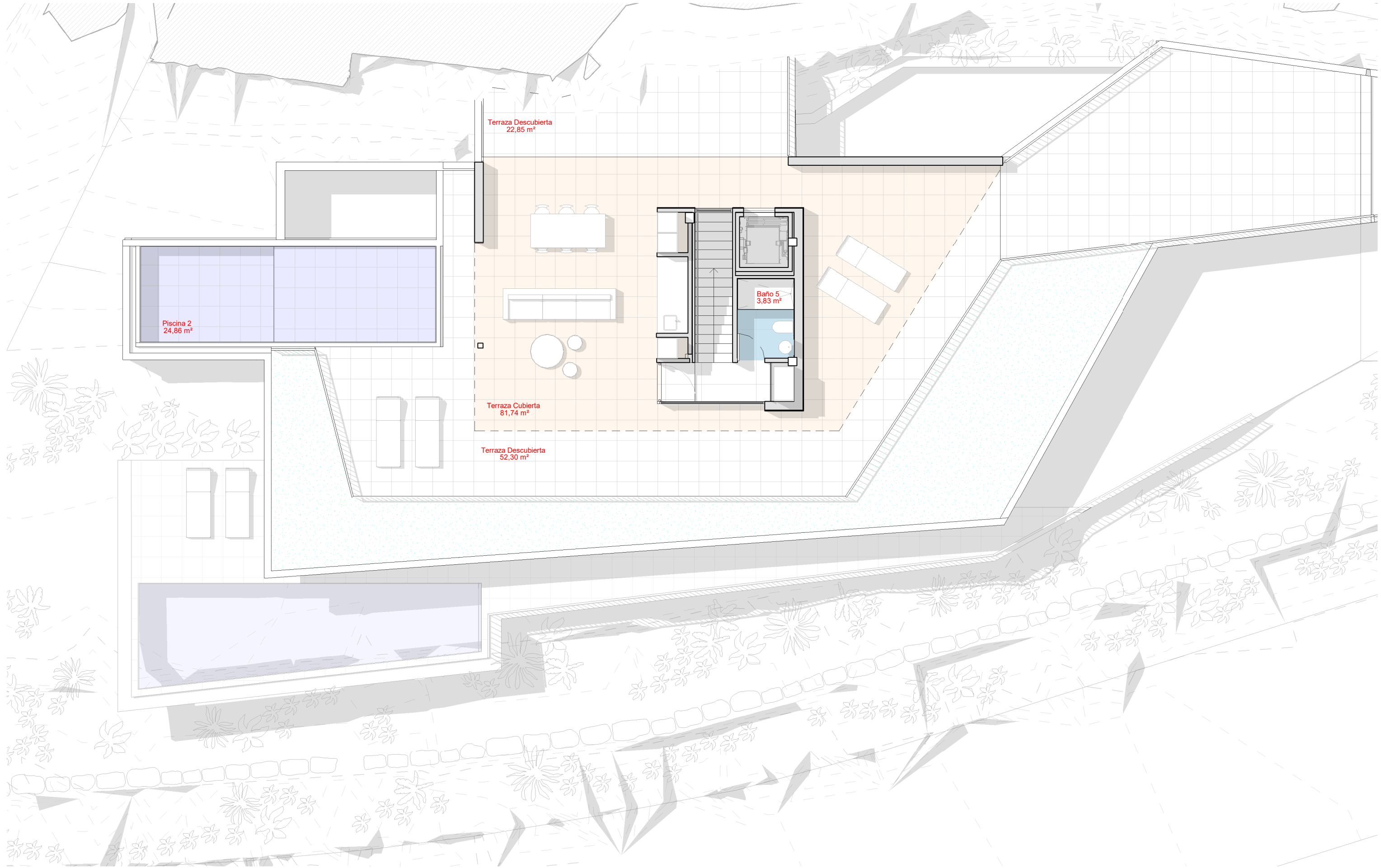
P01_Planta Primera_WEB 1 : 100
